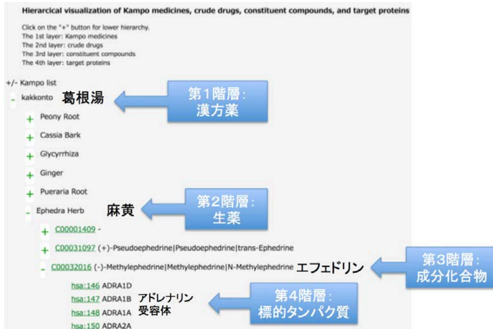
図1：漢方薬、生薬、成分化合物、標的タンパク質の階層関係を整備
