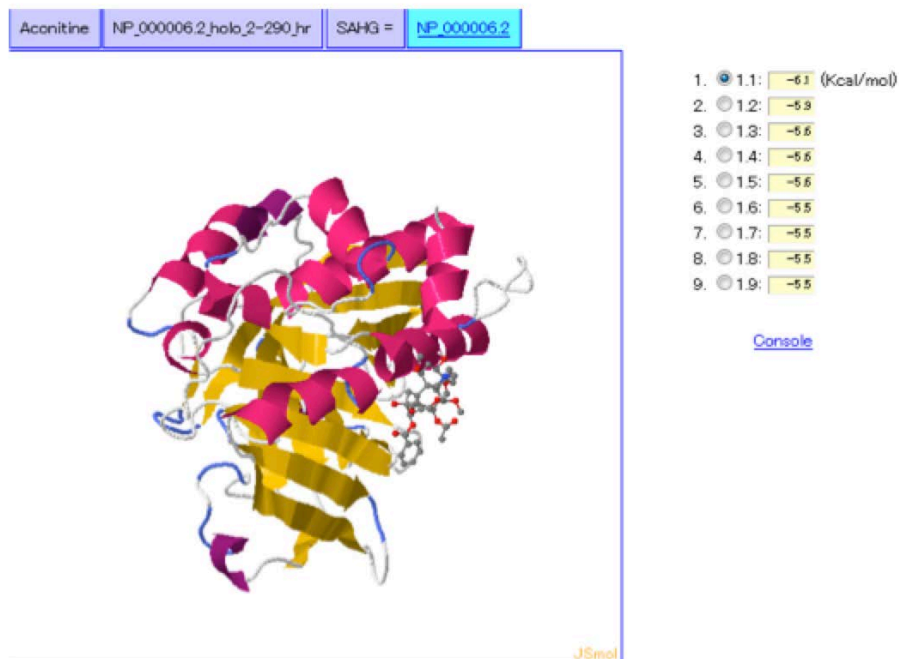
図3：漢方薬成分化合物とヒトのタンパク質の結合シミュレーション
