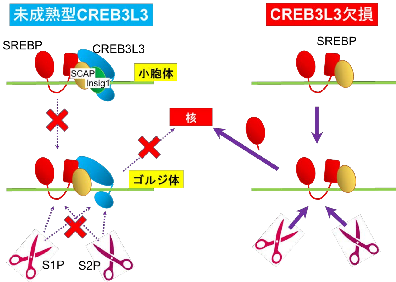
図1 CREB3L3 と SREBP の相互抑制メカニズム
